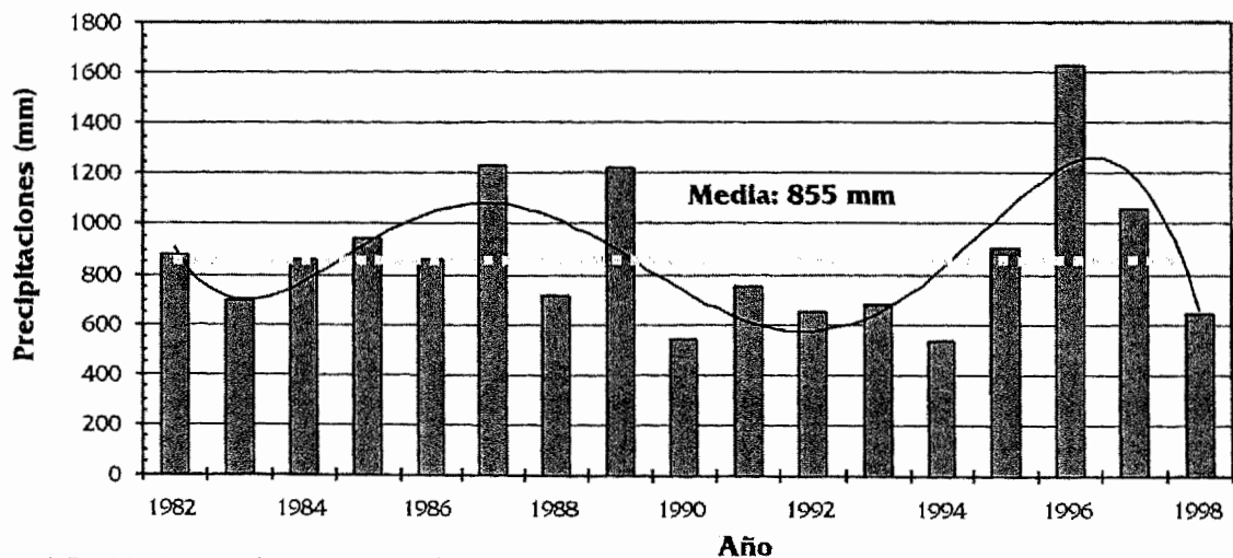
Figura 1. Precipitaciones totales anuales recogidas en la estación meteorológica del embalse de los Hurones, período 1982-1998
