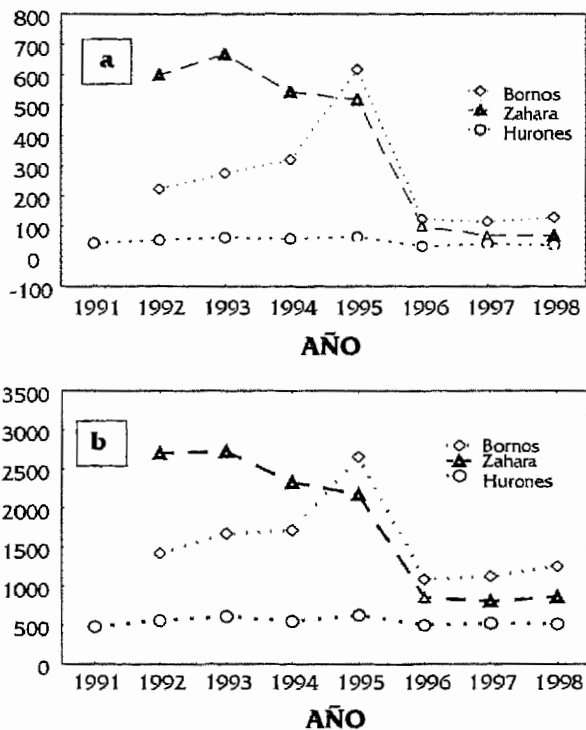
Figura 2. Evolución de los niveles medios de Cloruros (a) y Conductividad (b) en los embalses de las cuencas de los ríos Guadalete (Bornos y Zahara) y la del río Majaceite (Hurones).
