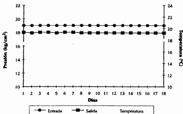
Figura 10: Evolución de los valores de presión y temperatura en el agua de entrada y presión del agua rechazado en el experimento con 25 mg/L de cloruro férrico.
