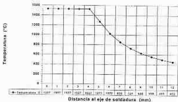
Figura 2. Ciclo térmico proceso S.M.A.W. en chapa gruesa.
