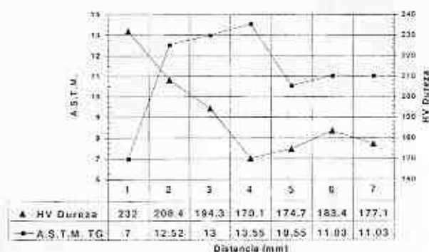
Figura 14. Dureza-tamaño de grano. Probeta P3T.
