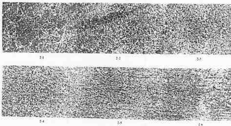
Figura 10. Mapa de la probeta P3T. Micrografías (2-1) - (2-6).
