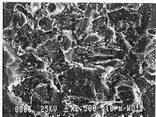
Figura 5. Región de cristalización. Probeta P3S x 2.500.
