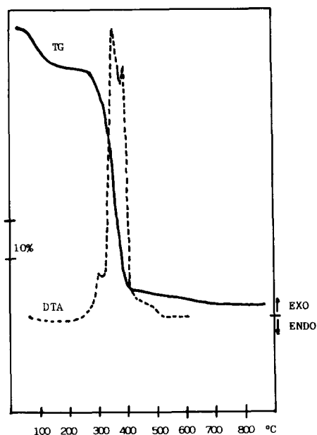
Fig. 1. DTA and TG curves for Na[Cr(EDTA)N 2 ] \cdot 2H 2 O.
